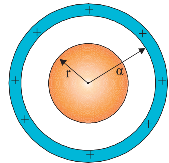
Σχ. 5.12 Η επιφάνεια Gauss είναι σφαίρα ομόκεντρη με το κέλυφος και με μικρότερη ακτίνα.
