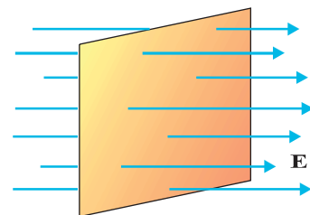
Σχ. 5.3 Η επιφάνεια είναι τοποθετημένη κάθετα στις δυναμικές γραμμές, ομογενούς ηλεκτρικού πεδίου.
