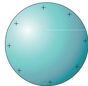
Σχ. 5.13 Όλο το φορτίο του σφαιρικού αγωγού βρίσκεται στην επιφάνειά του. Εξωτερικά ο αγωγός συμπεριφέρεται σαν όλο του το φορτίο να είναι συγκεντρωμένο στο κέντρο του (σαν σημειακό φορτίο). Στο εσωτερικό του αγωγού το πεδίο είναι μηδέν.
