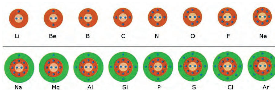
ΣΧΗΜΑ 2.2 Διαγραμματική απεικόνιση της κατανομής των ηλεκτρονίων σε στιβάδες (φλοιούς). Η ηλεκτρονιακή δομή των ατόμων, όπως φαίνεται στο σχήμα, εμφανίζει μια περιοδικότητα η οποία τελικά εκφράζεται στον περιοδικό πίνακα.
