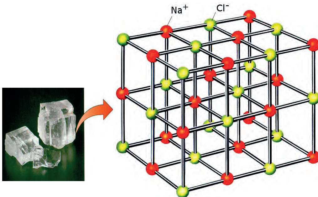
ΣΧΗΜΑ 1.7 Ο κρύσταλλος του NaCl συγκροτείται από ιόντα Na^+ και Cl^- .
