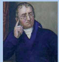
John Dalton 1766-1844
