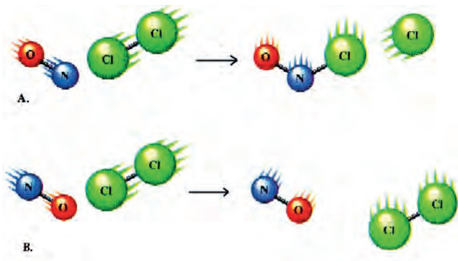
ΣΧΗΜΑ 3.8 Για να γίνει η αντίδραση \text{NO} + \text{Cl}_2 \rightarrow \text{NOCl} + \text{Cl} θα πρέπει τα αντιδρώντα μόρια να έχουν το σωστό προσανατολισμό και την κατάλληλη ταχύτητα (ενέργεια).
