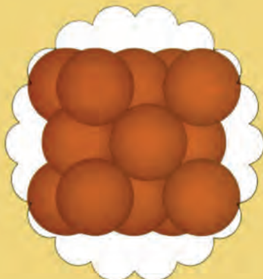
Άτομα
