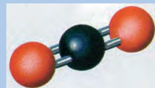
μόριο \text{CO}_2
