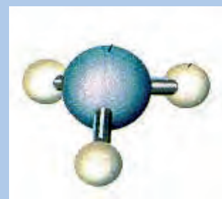
μόριο \text{NH}_3
