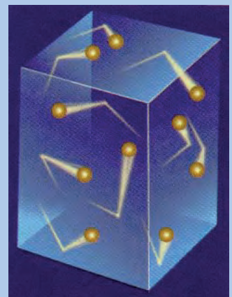
ΣΧΗΜΑ 4.6 Εικονική παρουσίαση του νόμου του Gay-Lussac. Η πίεση ενός αερίου είναι ανάλογος της απόλυτης θερμοκρασίας (με n, V σταθερά).
