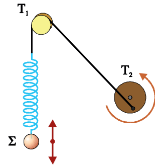
Το σώμα \Sigma εκτελεί εξαναγκασμένη ταλάντωση.
