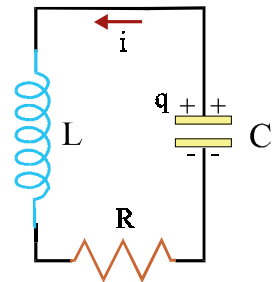
Κύκλωμα φθίνουσών ηλεκτρικών ταλαντώσεων. Σχήμα 1-22.
