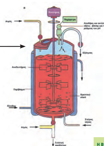
Εικόνα 7.3 α. Διαγραμματική απεικόνιση βιοαντιδραστήρα, όπου φαίνονται τα διάφορα τμήματά του, καθώς και οι συστασις αλλαγών των συνθηκών ζύμωσης β. Φωτογραφία βιοαντιδραστήρα.
