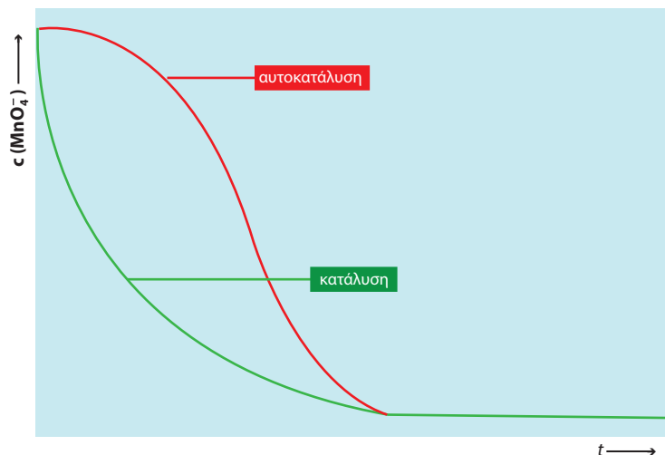
ΣΧΗΜΑ 3.6 Η καμπύλη της αντίδρασης στην κατάλυση και στην αυτοκατάλυση, με βάση την αντίδραση οξείδωσης του οξαλικού οξέος με υπερμαγγανικό κάλιο.
