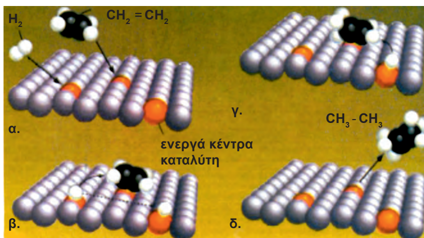
ΣΧΗΜΑ 3.8 Ερμηνεία της καταλυτικής δράσης του Ni στην αντίδραση \text{C}_2\text{H}_4(\text{g}) + \text{H}_2(\text{g}) \xrightarrow{\text{Ni(s)}} \text{C}_2\text{H}_6(\text{g}) με βάση τη θεωρία της προσρόφησης:
