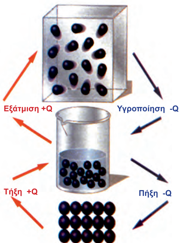
ΣΧΗΜΑ 1.7 Διαγραμματική απεικόνιση των τριών καταστάσεων της ύλης. Τα σωματίδια μπορεί να είναι μόρια ή ιόντα ή άτομα.
