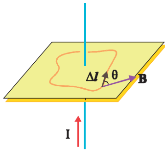
Σχ. 4.7 Το άθροισμά των γινομένων B\Delta l συνθ κατά μήκος οποιασδήποτε κλειστής διαδρομής που περικλείει το ρεύμα I είναι ίσο με \mu_0 I .
