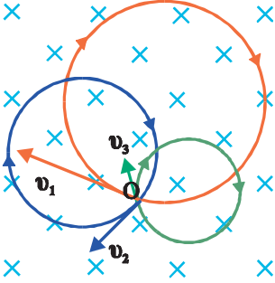
Σχ. 4.16 Τρία ηλεκτρόνια βάλλονται με διαφορετικές ταχύτητες κάθετα στις δυναμικές γραμμές ομογενούς μαγνητικού πεδίου στο σημείο Ο. Η ακτίνα της κυκλικής τροχιάς είναι ανάλογη της ταχύτητας. Η περίοδος είναι ίδια και στις τρεις περιπτώσεις.
