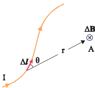
Σχ. 4.1 Το μαγνητικό πεδίο \Delta \mathbf{B} που δημιουργεί το τμήμα \Delta l του αγωγού στο σημείο A, είναι κάθετο στο επίπεδο του βιβλίου και με φορά από τον αναγνώστη προς το βιβλίο. Η φορά δηλώνεται με το \otimes .
