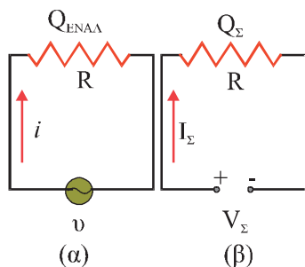
Σχ. 5.22 Αν η θερμότητα Q_Σ που παράγεται από το συνεχές ρεύμα I_Σ είναι ίση με τη θερμότητα Q_{ENAΛ} που παράγεται από το εναλλασσόμενο ρεύμα, τότε I_{ev} = I_Σ . Αν I_Σ = I_{ev} τότε V_Σ = V_{ev}
